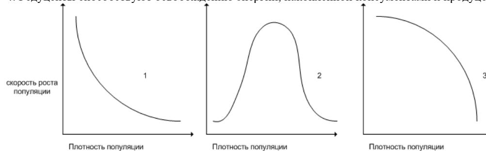
Рис.2. Популяционные волны
