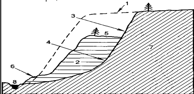
Рис. 3. Оползень
